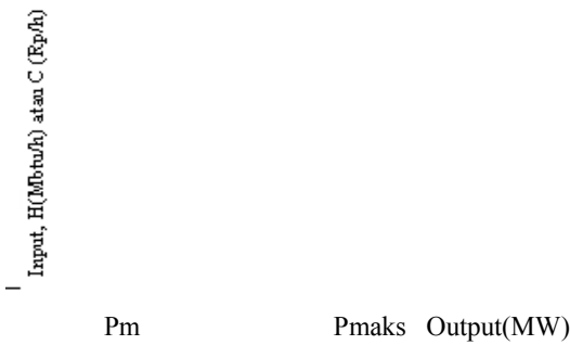
Gambar 1 Karakteristik input-output unit termal.
