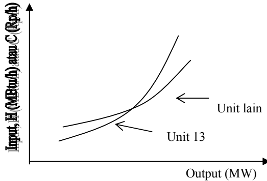
Gambar 6 Ilustrasi penomena pembebanan unit 13
