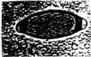
Telur T. trichiura . Telurnya panjangnya 50-54 \mu m dan lebarnya 22-23 \mu m, berwarna coklat kuningan sampai coklat kemerahan, berbentuk tong dengan kulit telur yang tebal dan tonjolan pada kedua kutub.
