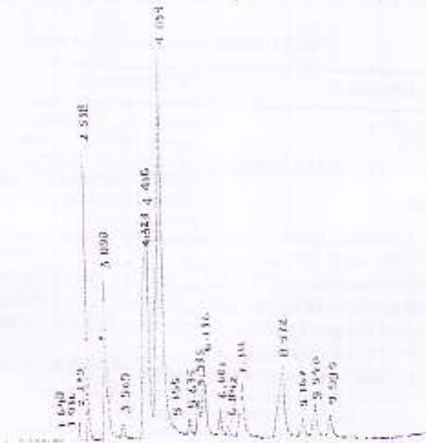
Gambar 1. Kromatogram minyak atsiri rhizoma Z. ottensii (kromatografi gas Hewlett Packard tipe 5890)
