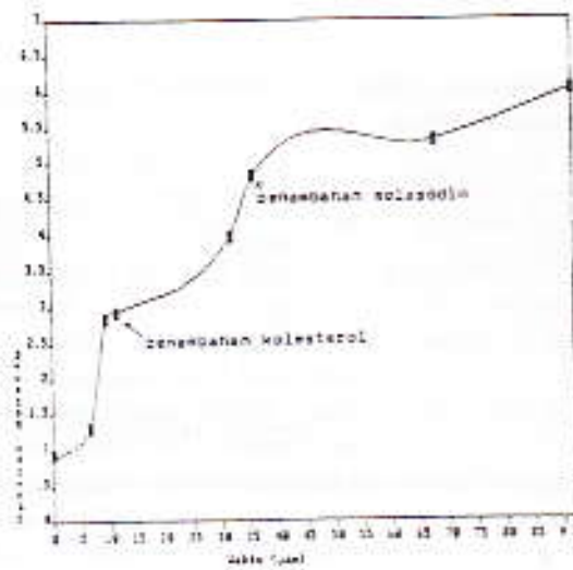
Gambar 1. Kurva Pertumbuhan bakteri Arthrobacter simplex dalam labu kock 500 ml.
