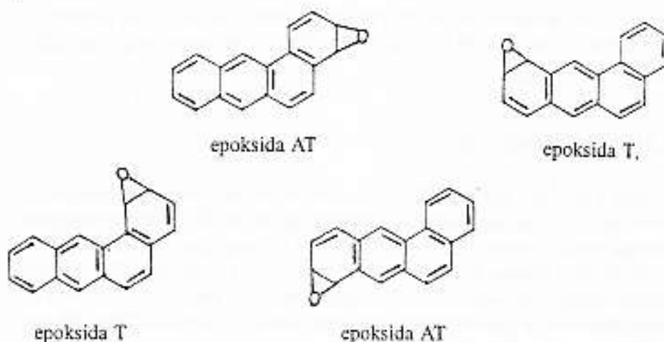
Skema 1. Benzo(a)antrasen mempunyai dua buah epoksida T dan dua buah epoksida AT
